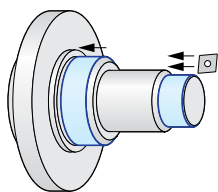
V_{max} : 0,15mm NMP AC8025P (150 pcs)
